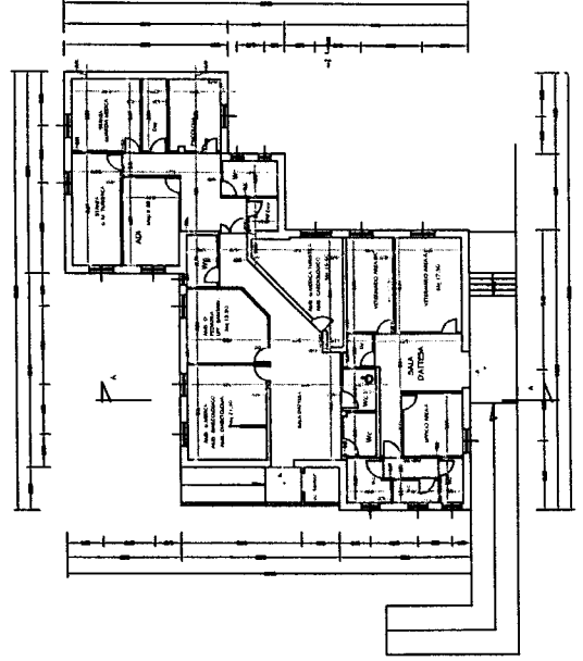
PIANTA PIANO TERRA SITUAZIONE IN PROGETTO
